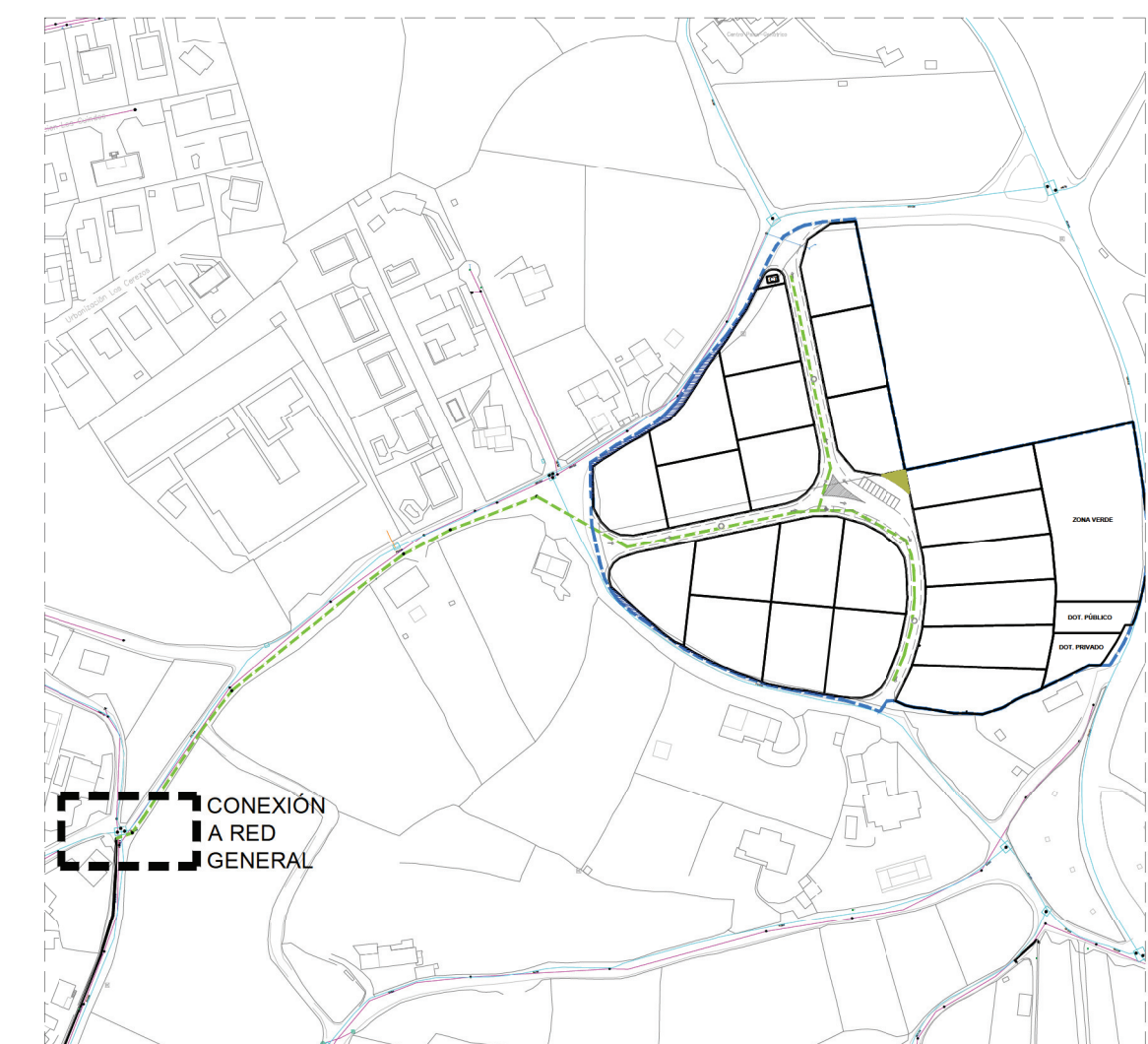
PROPUESTA 1 RECOGIDA DE AGUAS PLUVIALES: CONEXIÓN A RED GENERAL EXISTENTE EN CAMINO MONTEVIENTO
