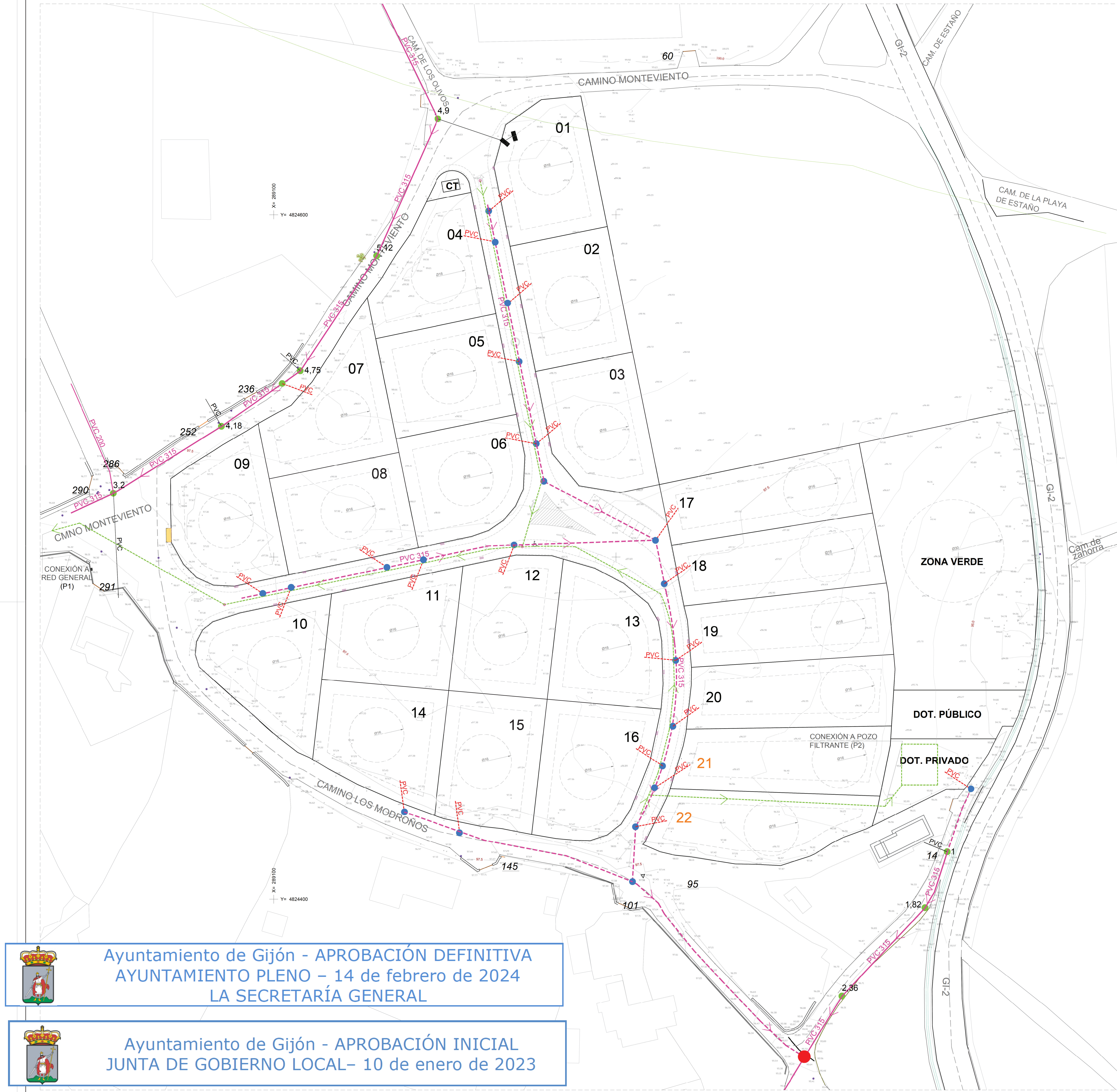
PROPUESTA 1 RECOGIDA DE AGUAS PLUVIALES: CONEXIÓN A RED GENERAL EXISTENTE EN CAMINO MONTEVIENTO
